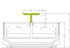
WNE/WDE - 01/03/04/06/07 - ONE LEVEL SUPERSTRUCTURE
