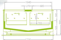
WNE/WDE-06
