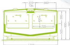
WNE/WDE-06-SLIDE
